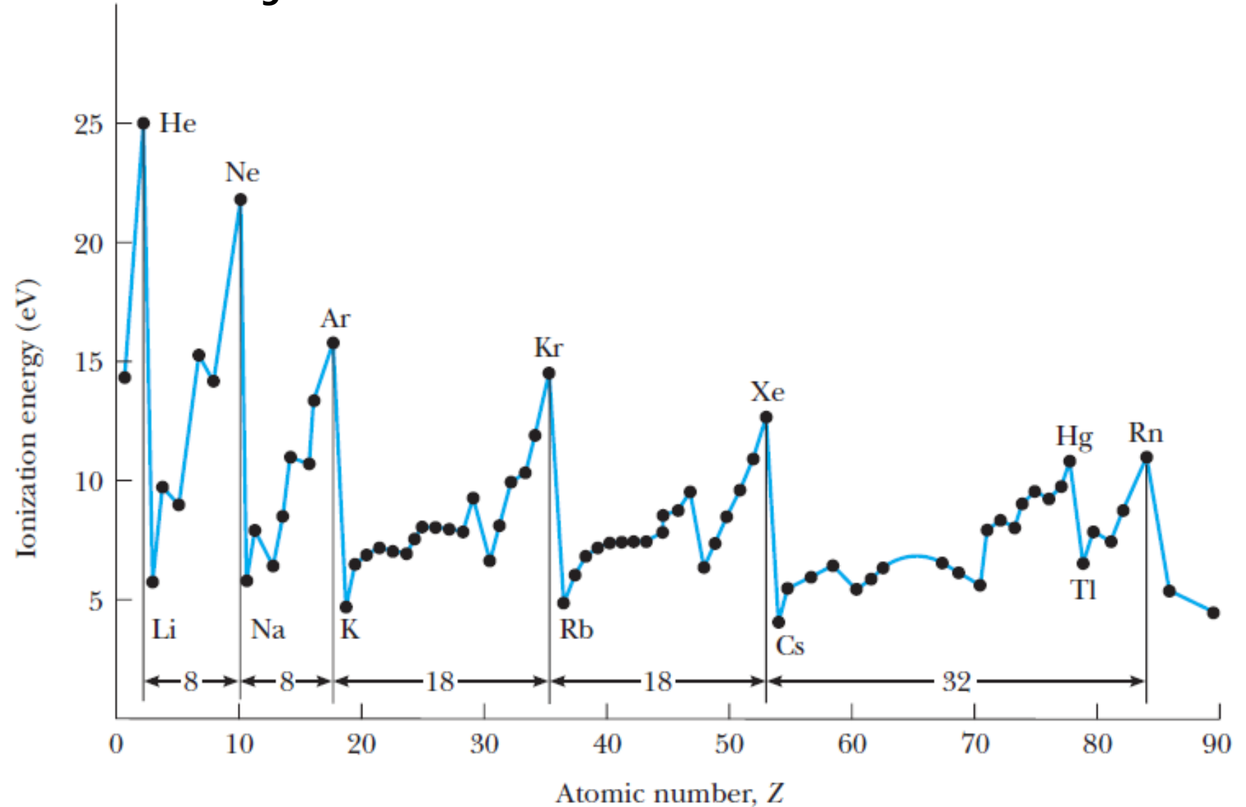
Energía de ionización vs número atómico
